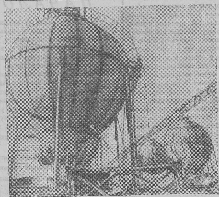
НА СНИМКЕ: монтаж газовых резервуаров. Фото МТИ—ТАСС
