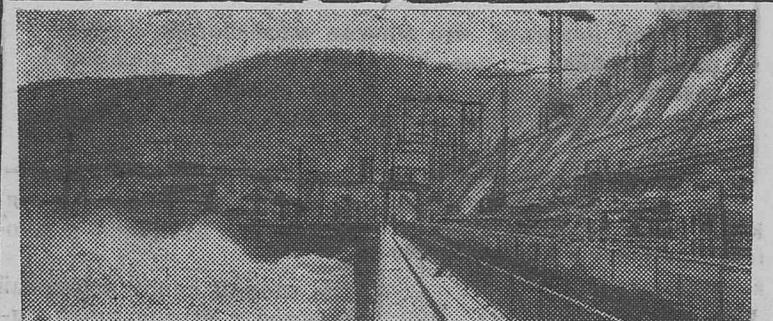
Дивногорск. Панорама строительства Красноярской ГЭС с нижнего бьефа. Фото Ю. Бармина. Фотохроника ТАСС
