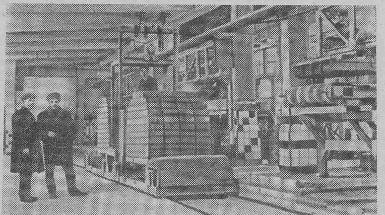
Воронежский завод силикатного кирпича. Цех, в котором установлены новые автоматы для съема с револьверного пресса и укладки на запарочную вагонетку силикатного кирпича-сырца. Фото В. Кожевникова. Фотохроника ТАСС
